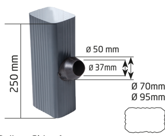
7016 Balkon Gider Aparatı Balcony Drain Fitting
