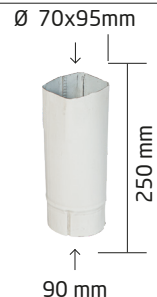
9002 Redüksiyon Köşeliden Yuvarlağa Geçiş Reducing
