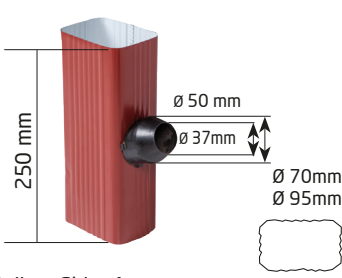
3009 Balkon Gider Aparatı Balcony Drain Fitting
