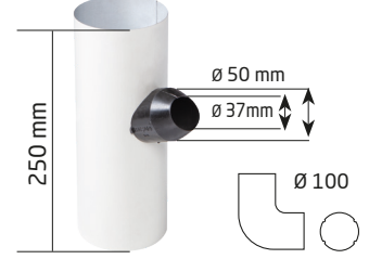
9002 Balkon Gider Aparatı Balcony Drain Apparatus
