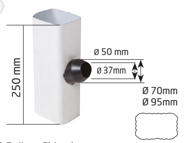
9002 Balkon Gider Aparatı Balcony Drain Fitting
