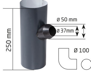
7016 Balkon Gider Aparatı Balcony Drain Apparatus
